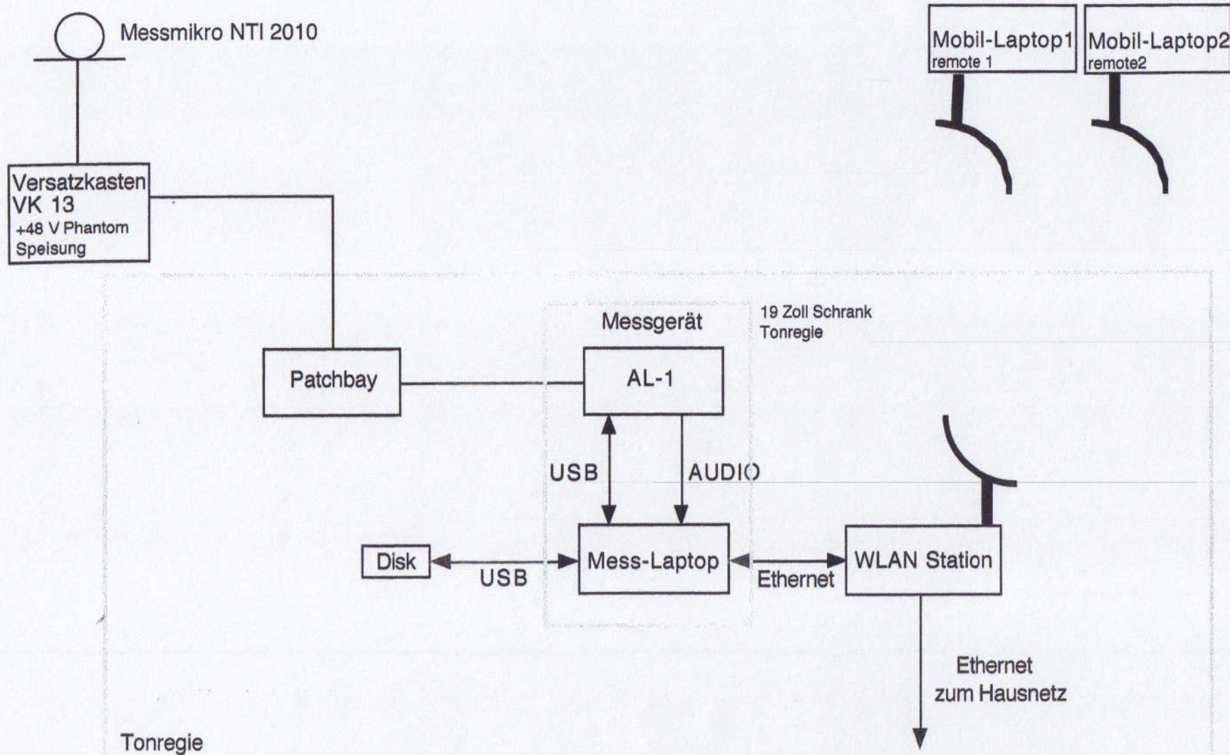
Blockschaltbild Pegelmesseinrichtung Hebbel Theater
